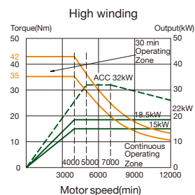
Fanuc α L8/15000i (Vc-205)
