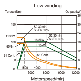
Fanuc α i15/12000 (Vc-305)
